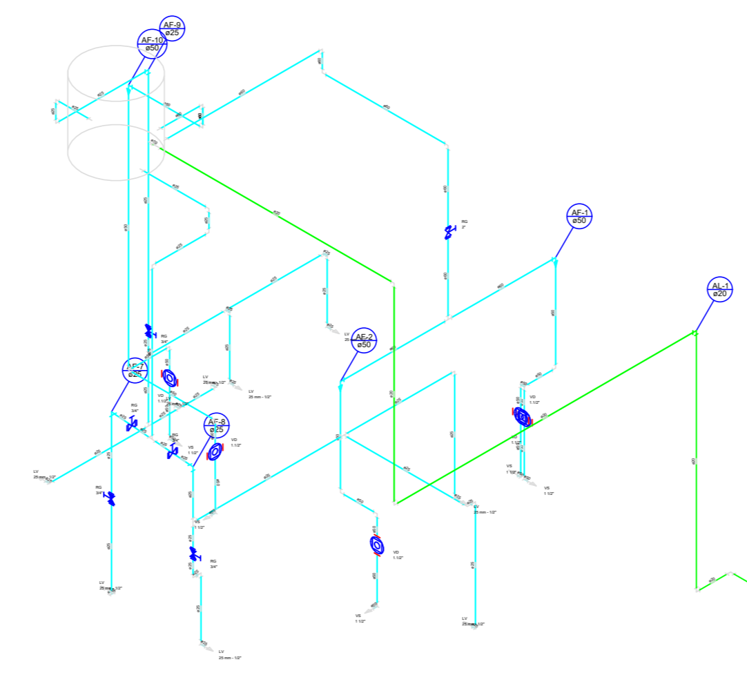
ESQUEMA ISOMÉTRICO DE ÁGUA Escala: 5/ ESCALA
